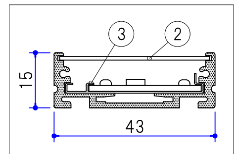
A-A' 断面図 (1/1)
