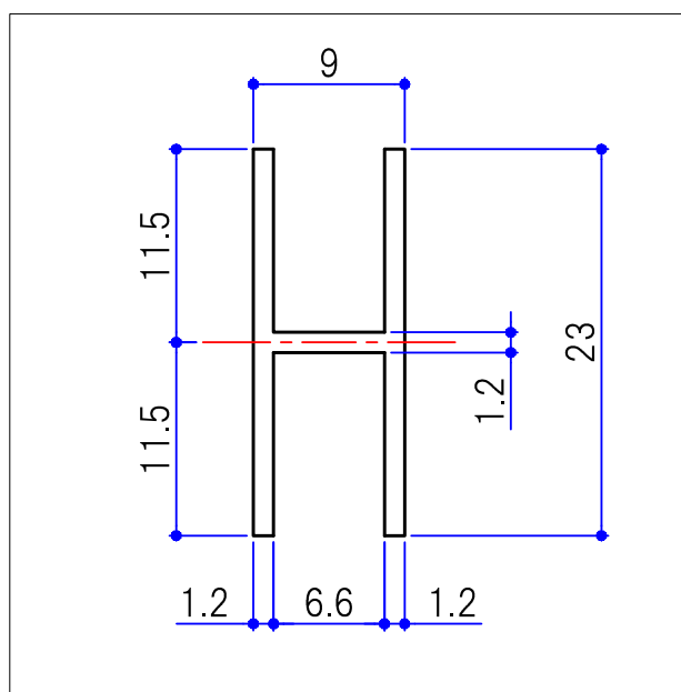
断面詳細図 (2/1)
