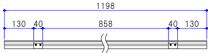
② 金具取付位置参照図 (1/8)
