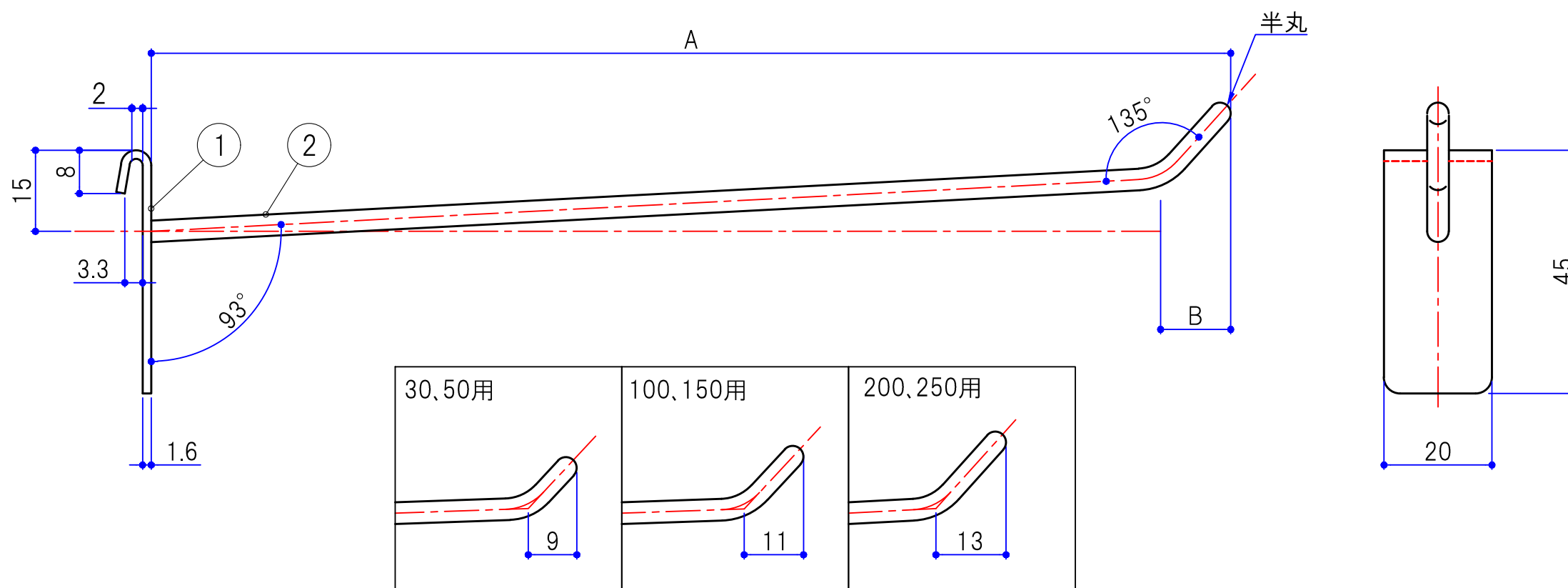
先端寸法図
