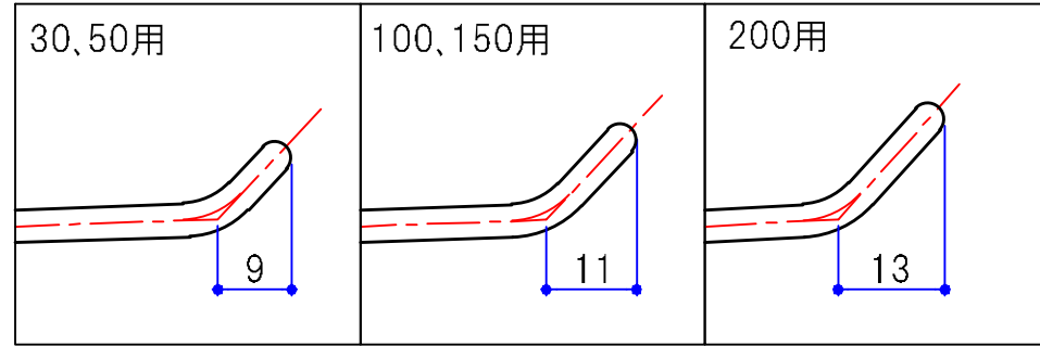
先端寸法図
