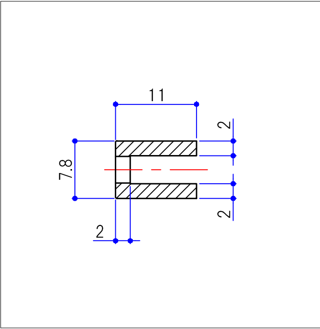
A-A断面詳細図 (2/1)
