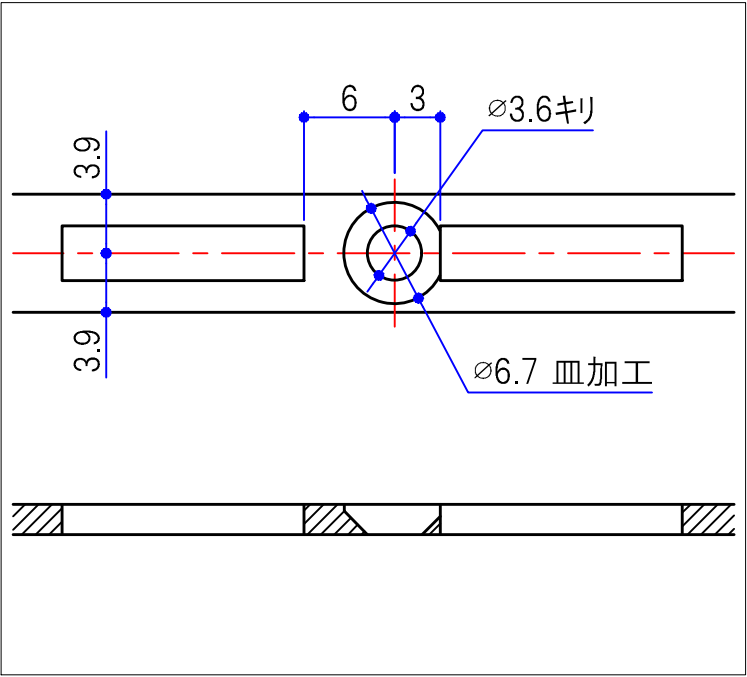
B-B断面 詳細図 (2/1)
