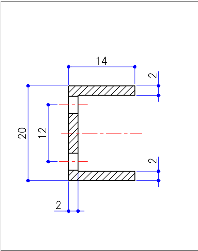
A-A断面詳細図 (2/1)
