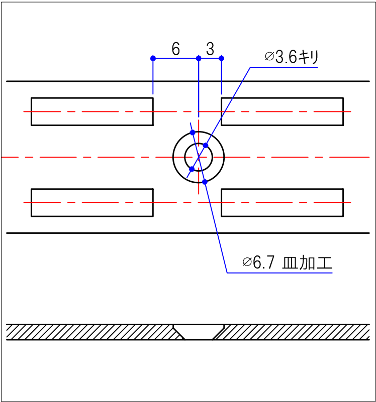
B-B断面 詳細図 (2/1)
