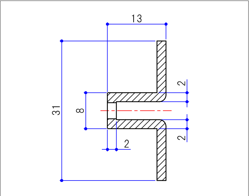
A-A 断面詳細図 (2/1)
