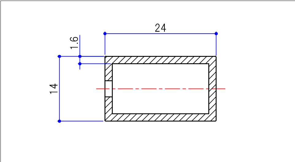
A-A 断面詳細図 (2/1)
