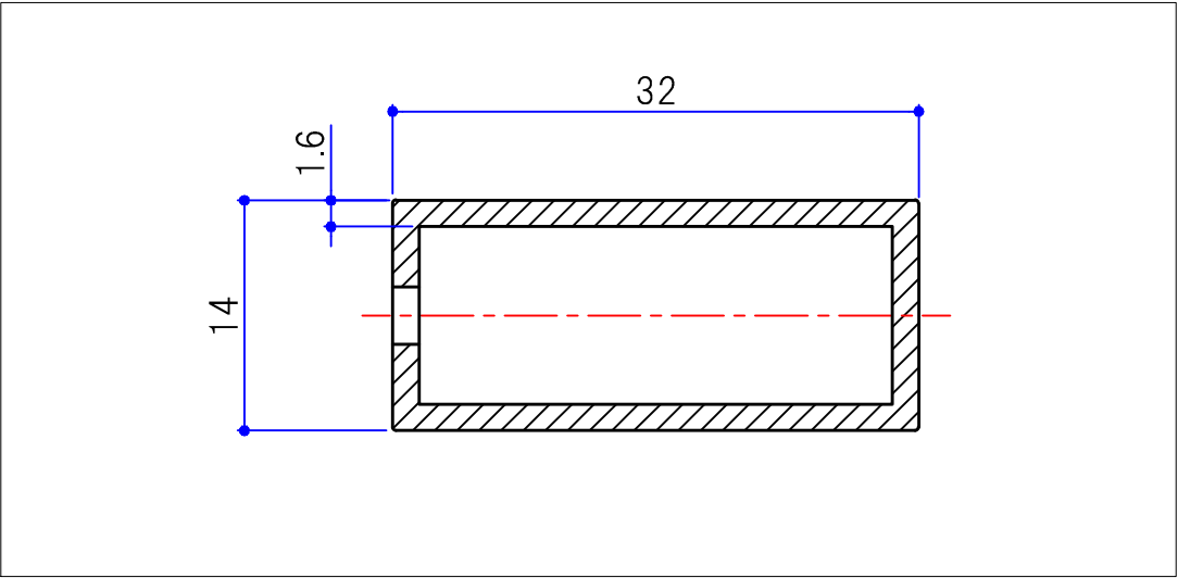
A-A 断面詳細図 (2/1)
