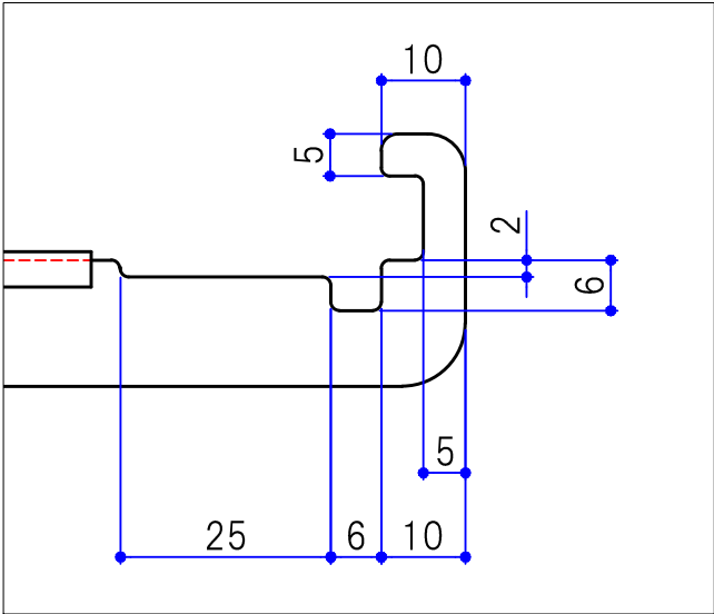
爪部詳細図 (1/1)
