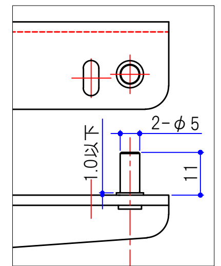
かしめダボ付き図 (1/1)
