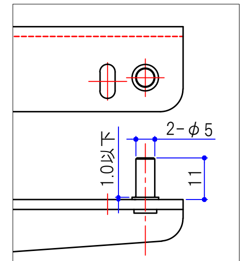
かしめダボ付き図 (1/1)
