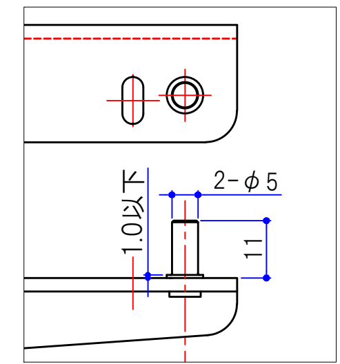
かしめダボ付き図 (1/1)
