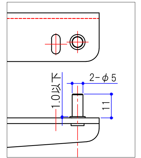
かしめダボ付き図 (1/1)
