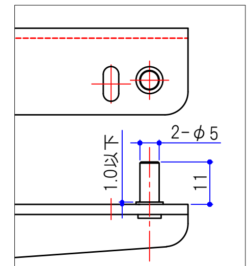
かしめダボ付き図 (1/1)
