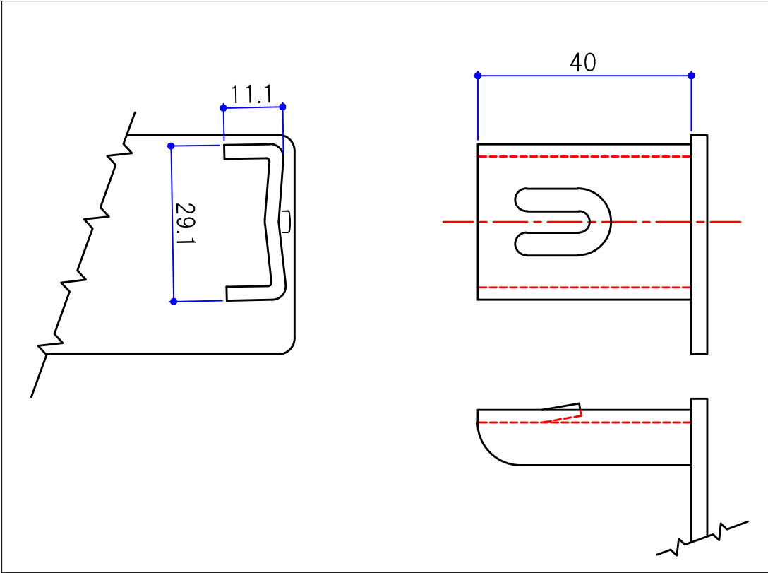
B部詳細図 (1/1)
