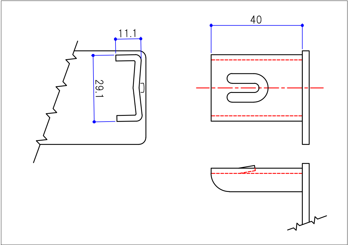
B部詳細図 (1/1)
