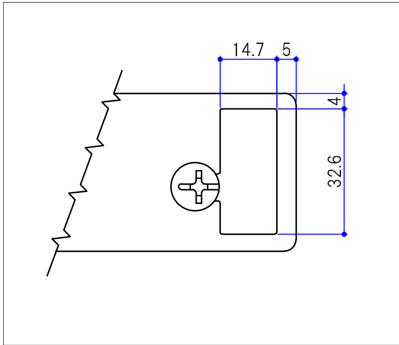
B部詳細図 (1/1)
