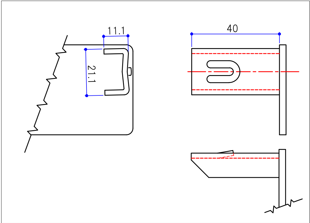
B部詳細図 (1/1)
