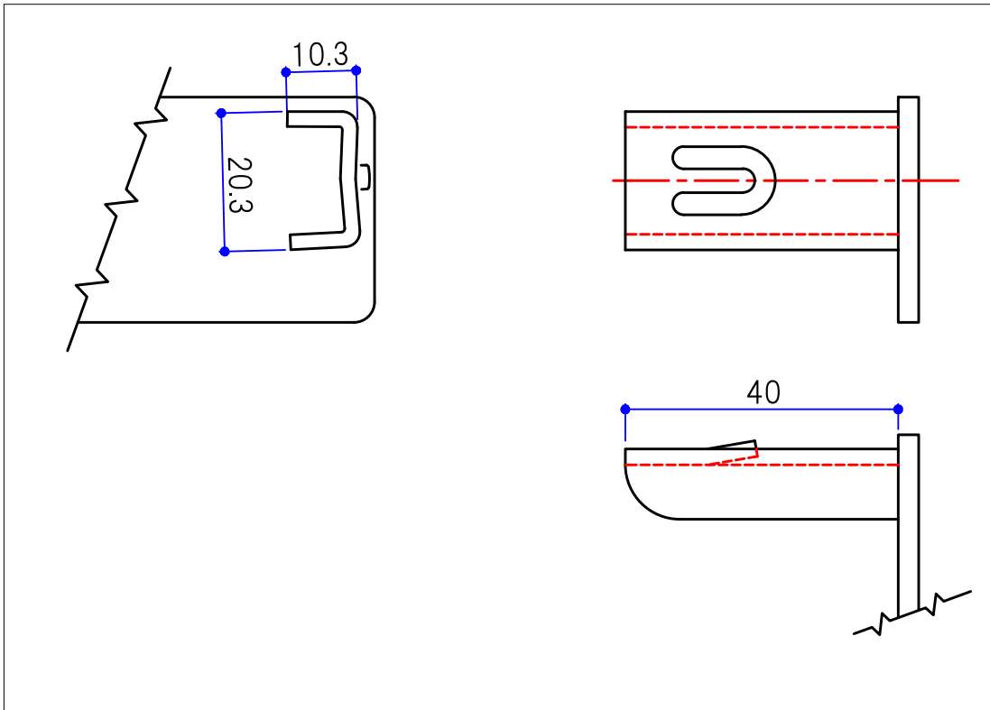
B部詳細図 (1/1)
