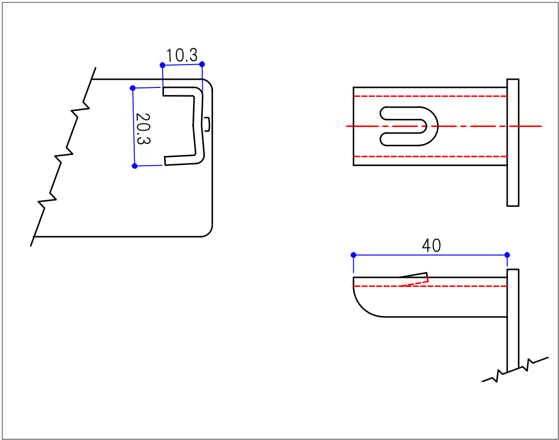
B部詳細図 (1/1)
