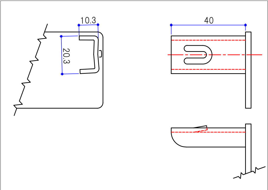
B部詳細図 (1/1)
