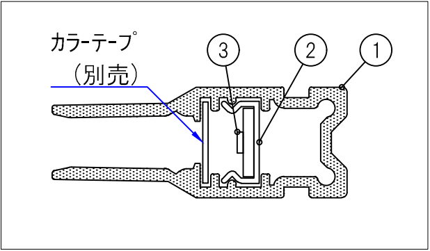
A-A 断面図 (2/1)
