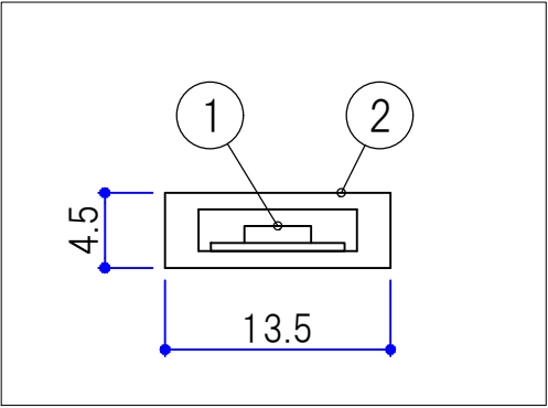
断面図 (2/1)
