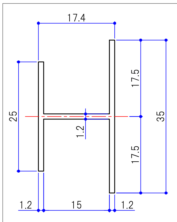
断面詳細図 (2/1)
