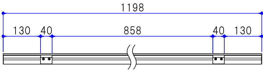
③ 金具取付位置参照図 (1/8)
