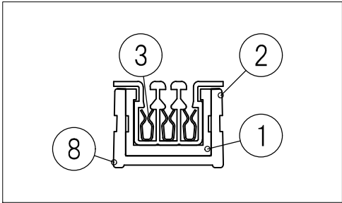
A-A 断面図 (1/1)
