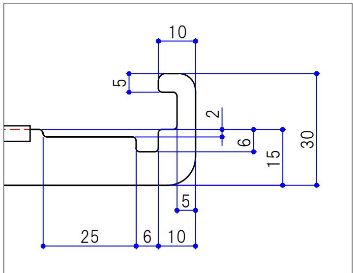
爪部詳細図 (1/1)
