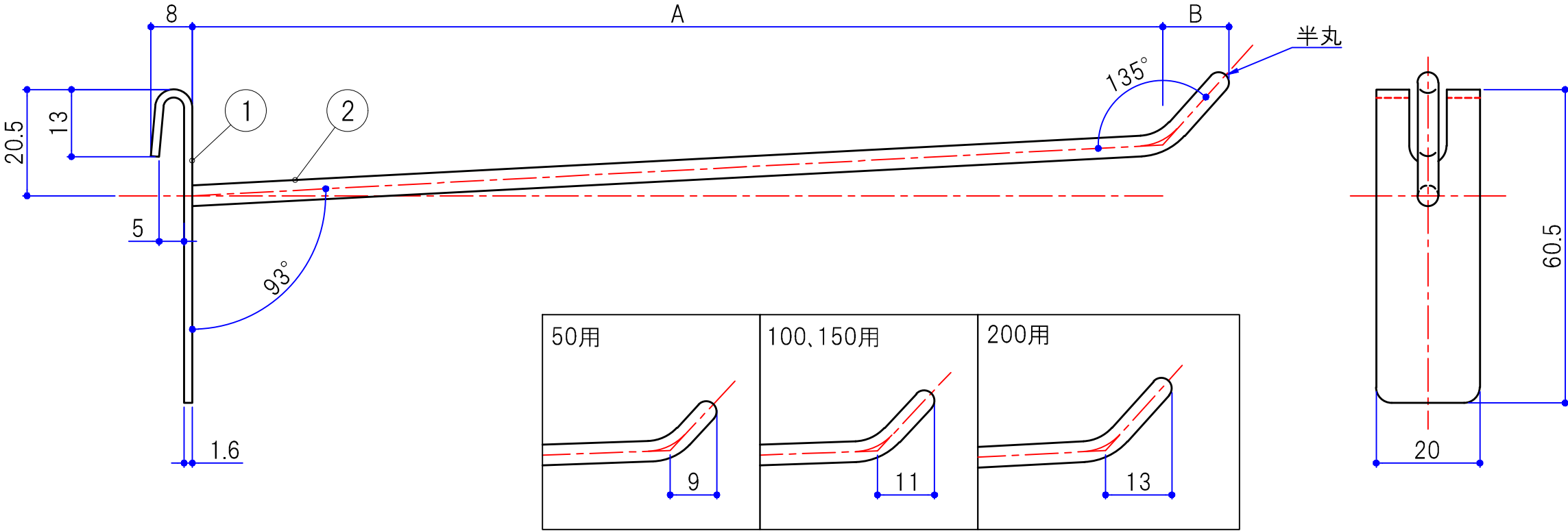
先端寸法図
