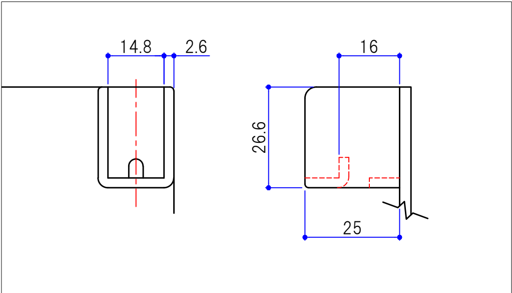
金具詳細図
