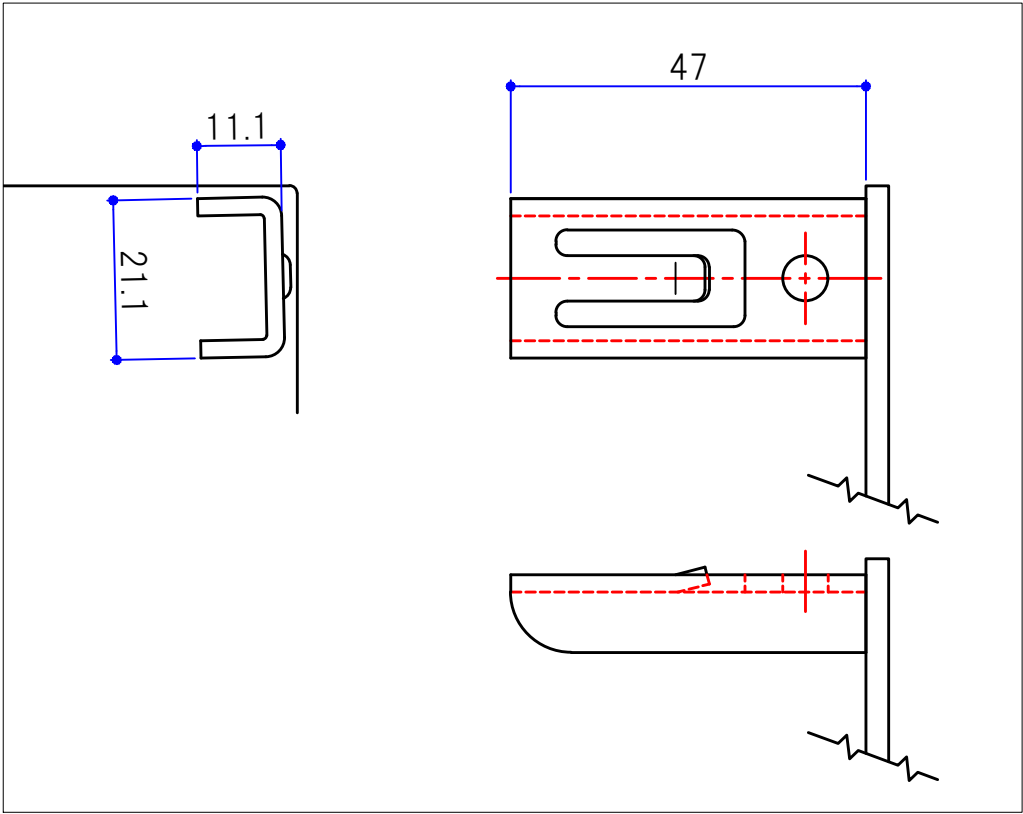
金具詳細図
