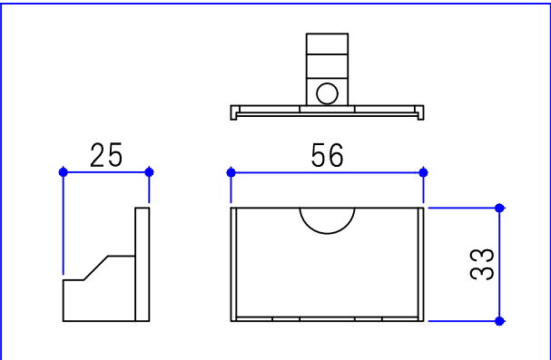
③ カードホルダー(固定式)W50×H30
