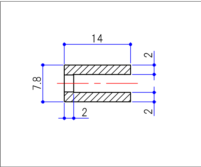
A-A 断面詳細図 (2/1)
