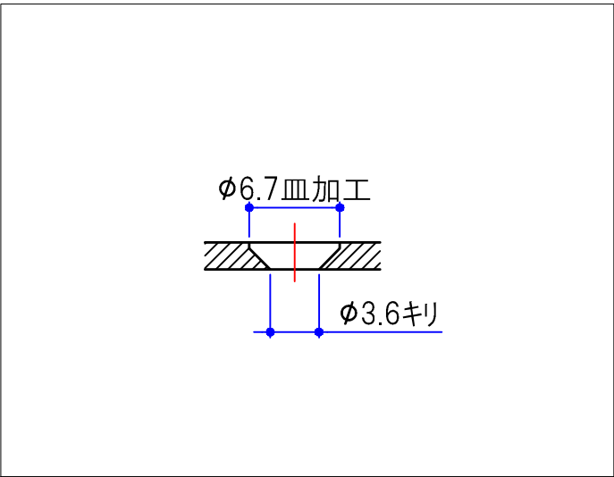
B-B 断面詳細図 (2/1)
