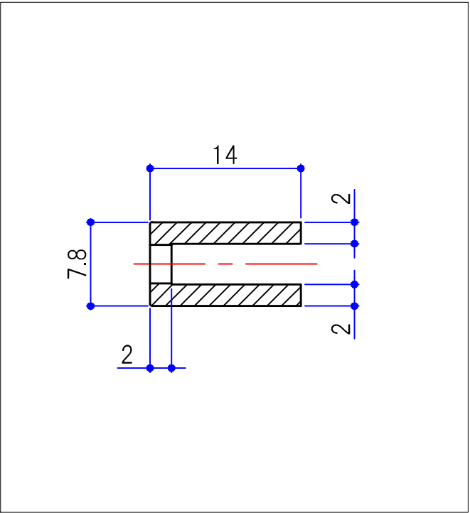
A-A断面詳細図 (2/1)
