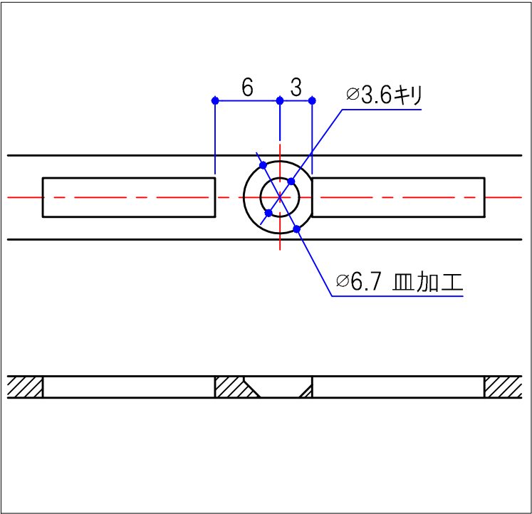
B-B断面 詳細図 (2/1)
