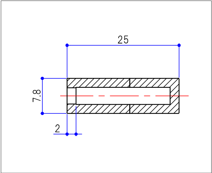
A-A 断面詳細図 (2/1)
