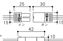
S S コネクタ仕様図
