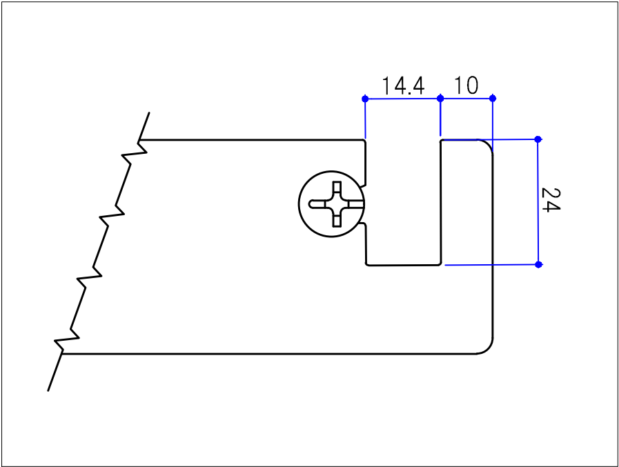
B部詳細図 (1/1)
