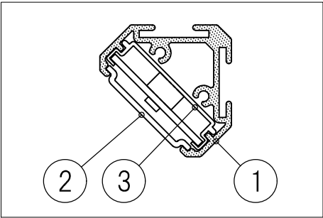
A-A 断面図 (1/1)
