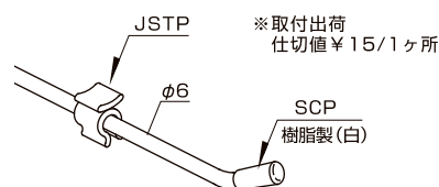
フック用樹脂ストッパーφ6用 (梱包数 100)
