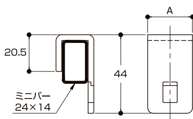
ミニバー 24×14 用 溶接用フック金具 (生地)
