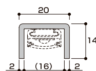
HKB142断面
