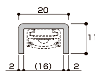
HKB112断面
