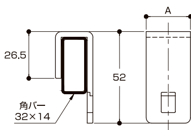
角バー 32×14 用 溶接用フック金具 (生地)
