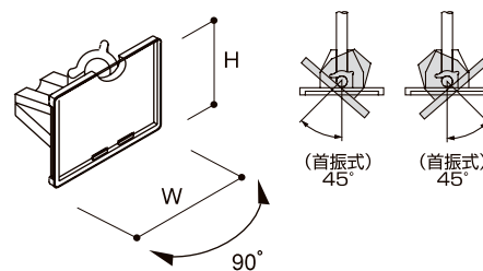
カードホルダー (首振り式) φ6 用
